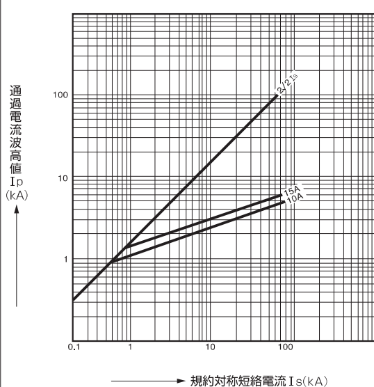
限流特性
