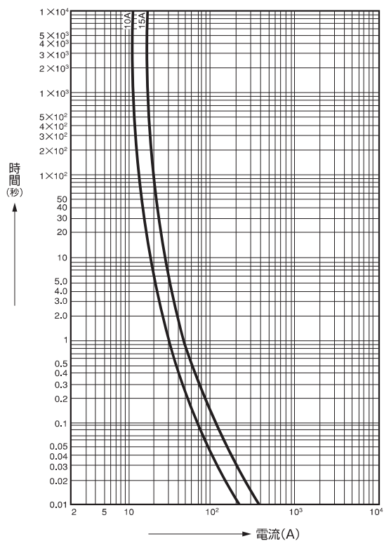
許容時間 — 電流特性
