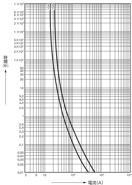
溶断時間 — 電流特性
