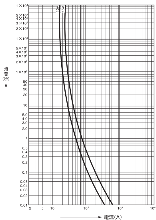
動作時間 — 電流特性
