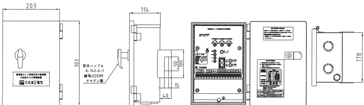
機種例：RDGV-3（ステンレス製） RDGV-4（ステンレス製）
