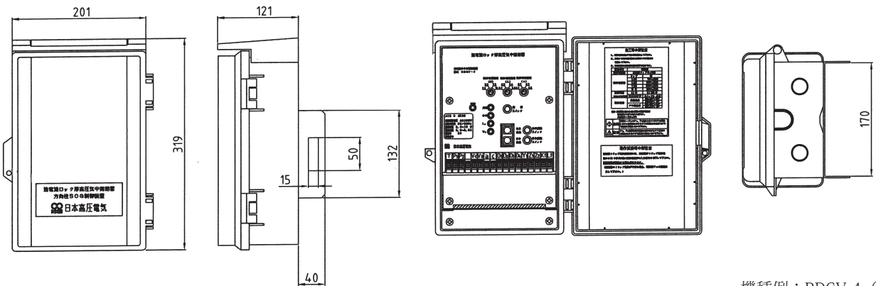
機種例：RDGV-4（樹脂製）
