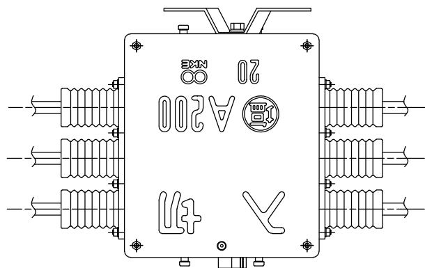
底面図
