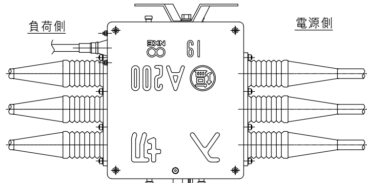
底面図
