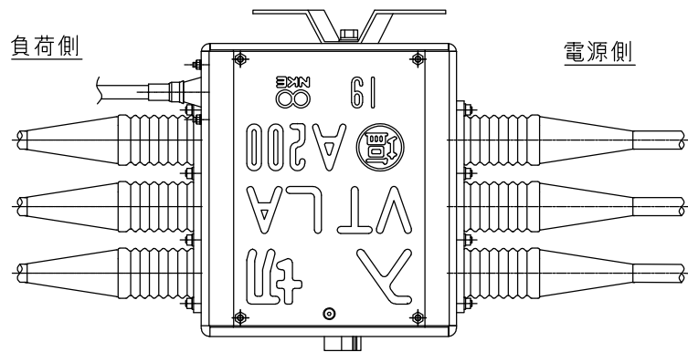
底面図
