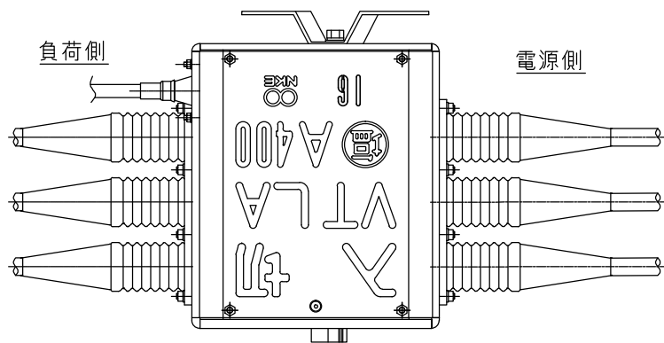
底面図
