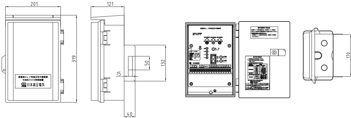
機種例：RDGV-3（樹脂製）
