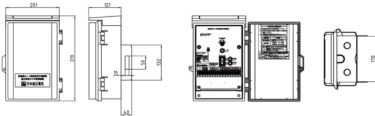
機種例：RASV-3（樹脂製）
