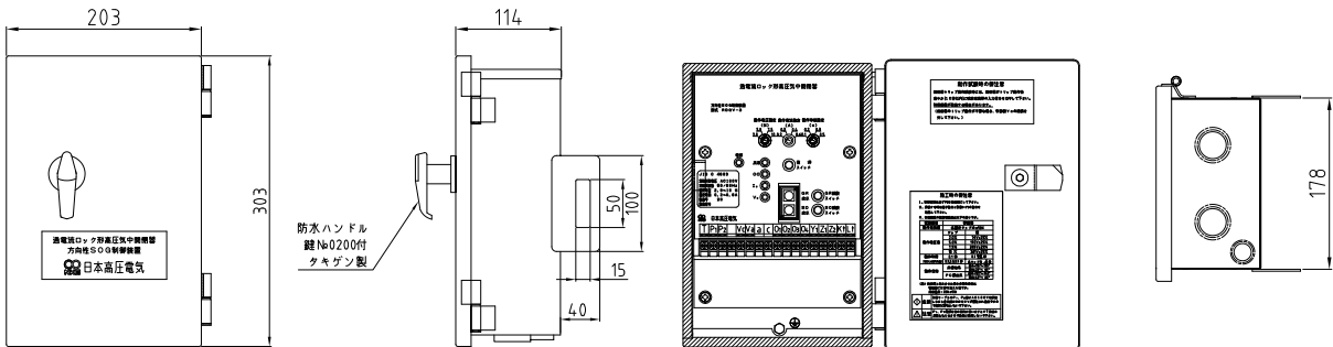
機種例：RDGV-3（ステンレス製）
