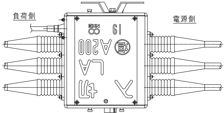
底面図
