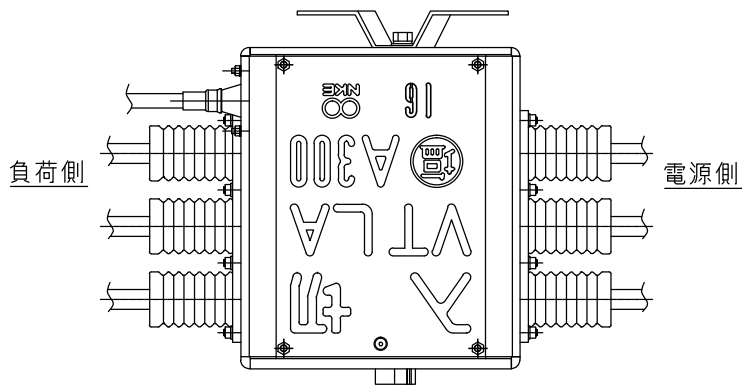
底面図
